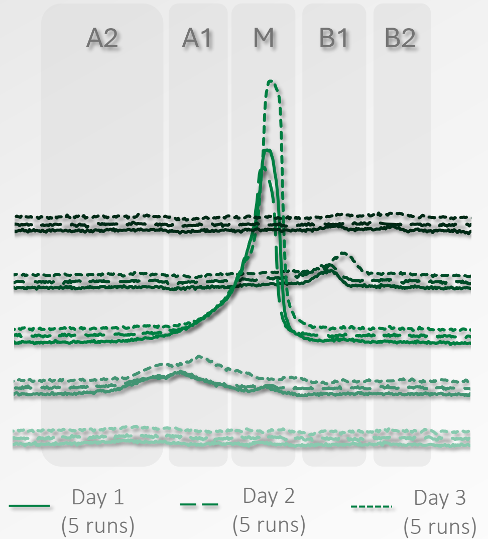
icIEF Fractionation
