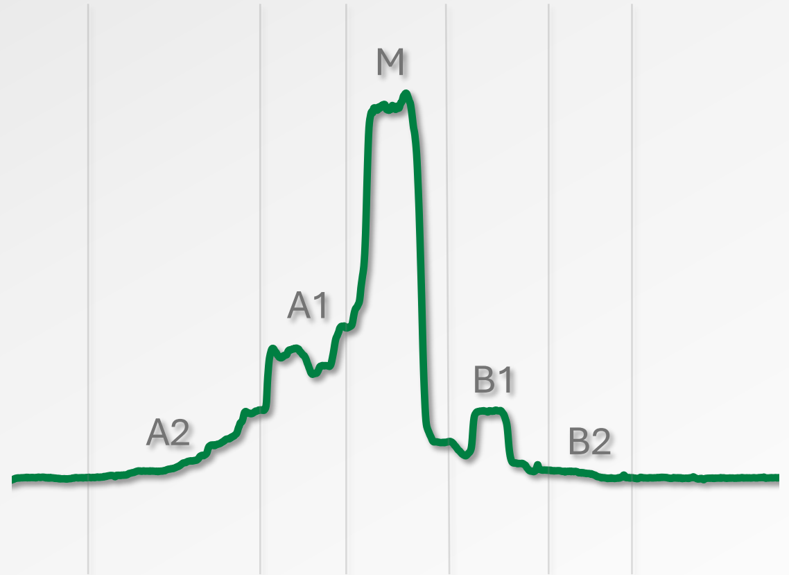
icIEF Fractionation
